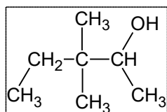
(15) 3,3-diméthylpentan-2-ol
