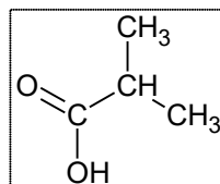
(23) Acide méthylpropanoïque
