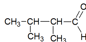
(19) 2,3-diméthylbutanal
