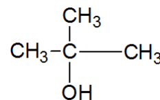
(8) méthylpropan-2-ol
