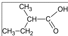
(11) Acide 2-méthylbutanoïque
