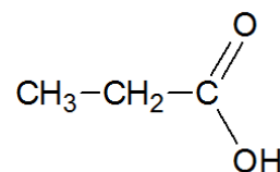
(4) acide propanoïque
