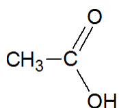
(13) acide éthanoïque
