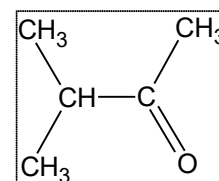
(17) Méthylbutanone
