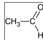
(5) éthanal
