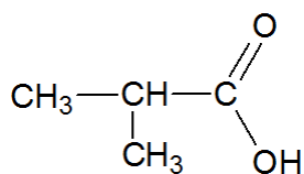
(17) acide méthylpropanoïque
