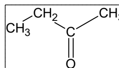
(16) Butanone
