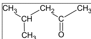
(8) 4-méthylpentan-2-one
