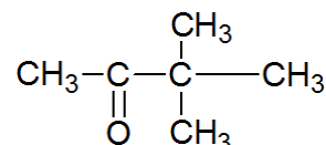
(16) diméthylbutanone
