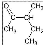
(20) 3-méthylpentan-2-one
