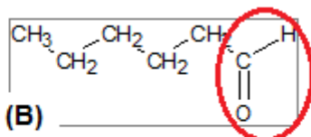
aldéhyde : hexanal
