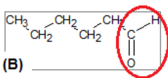
aldéhyde : hexanal
