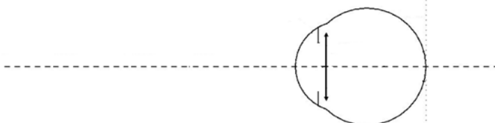
Fig (g) :Un œil hypermétrope corrigé par des lunettes regarde un objet situé à l'infini
